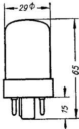
Kolbenabmessungen
