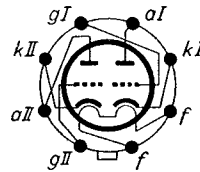
Sockelschaltenschema
